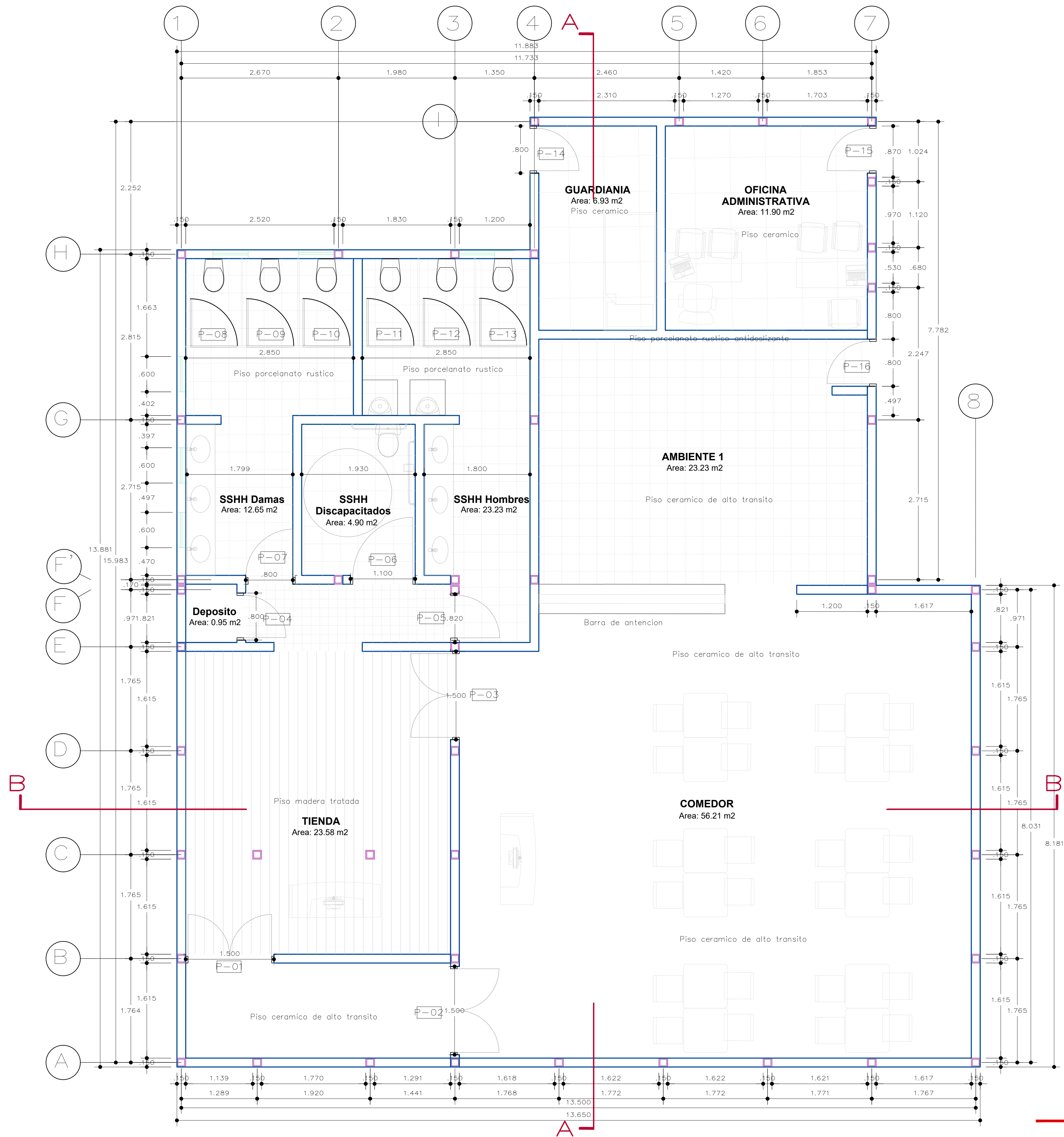
PLANO DE CAFETERIA
