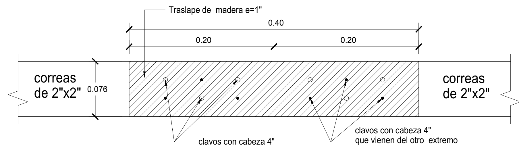
EMPALME DE CORREAS (Escala : 1/2)
