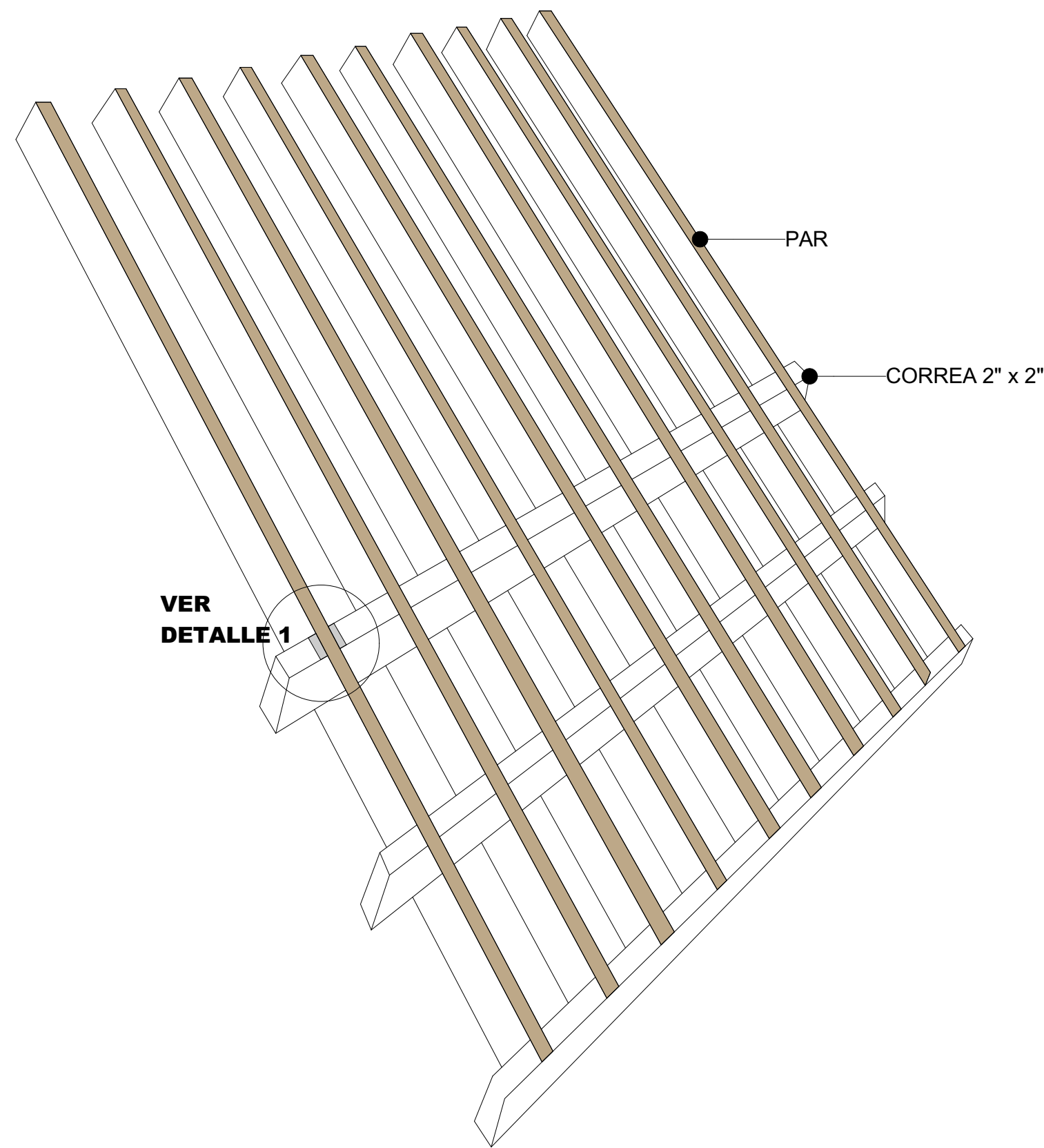
DETALLE ESTRUCTURAL DE CUBIERTA
