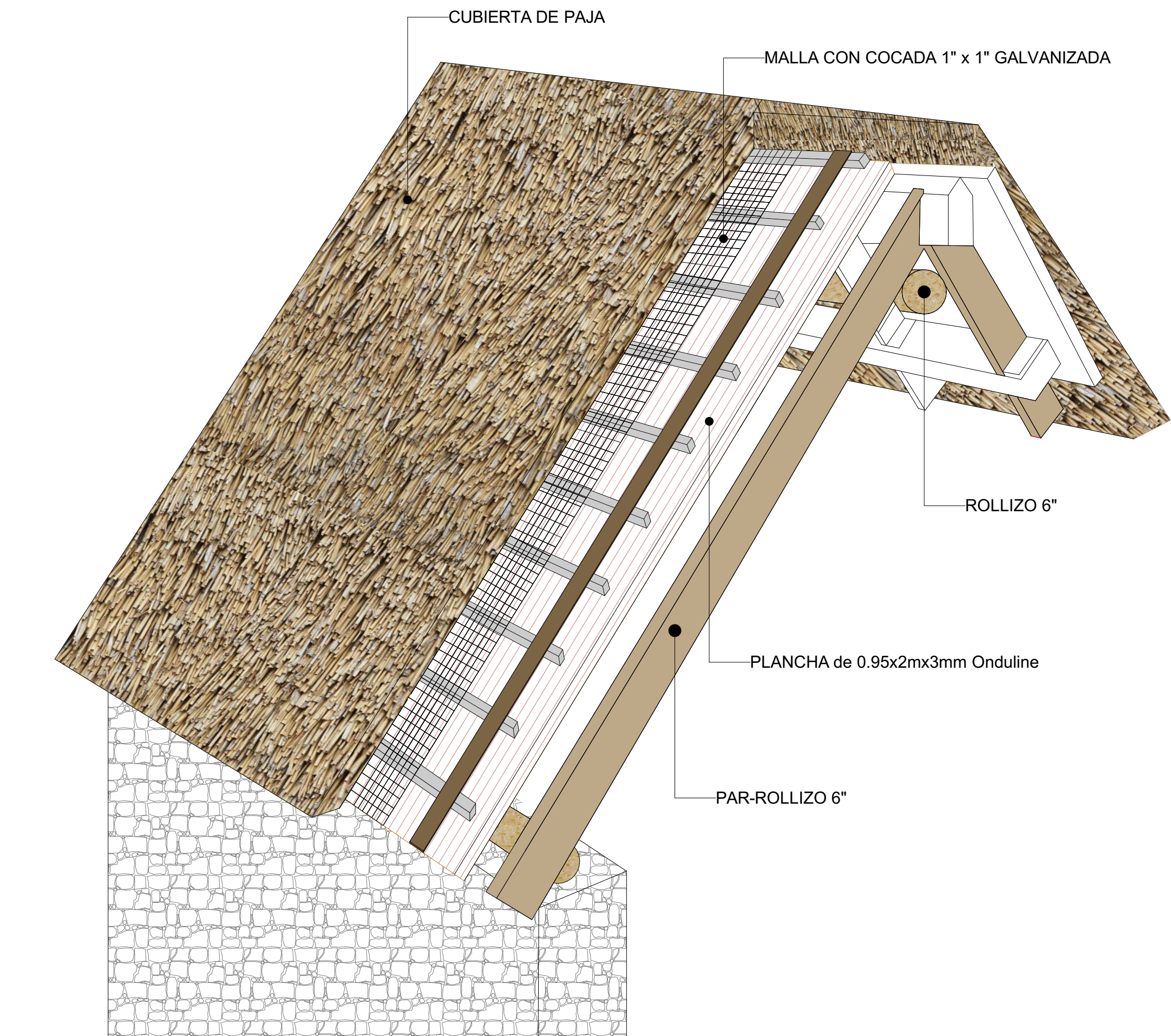
DETALLE ESTRUCTURAL DE CUBIERTA
