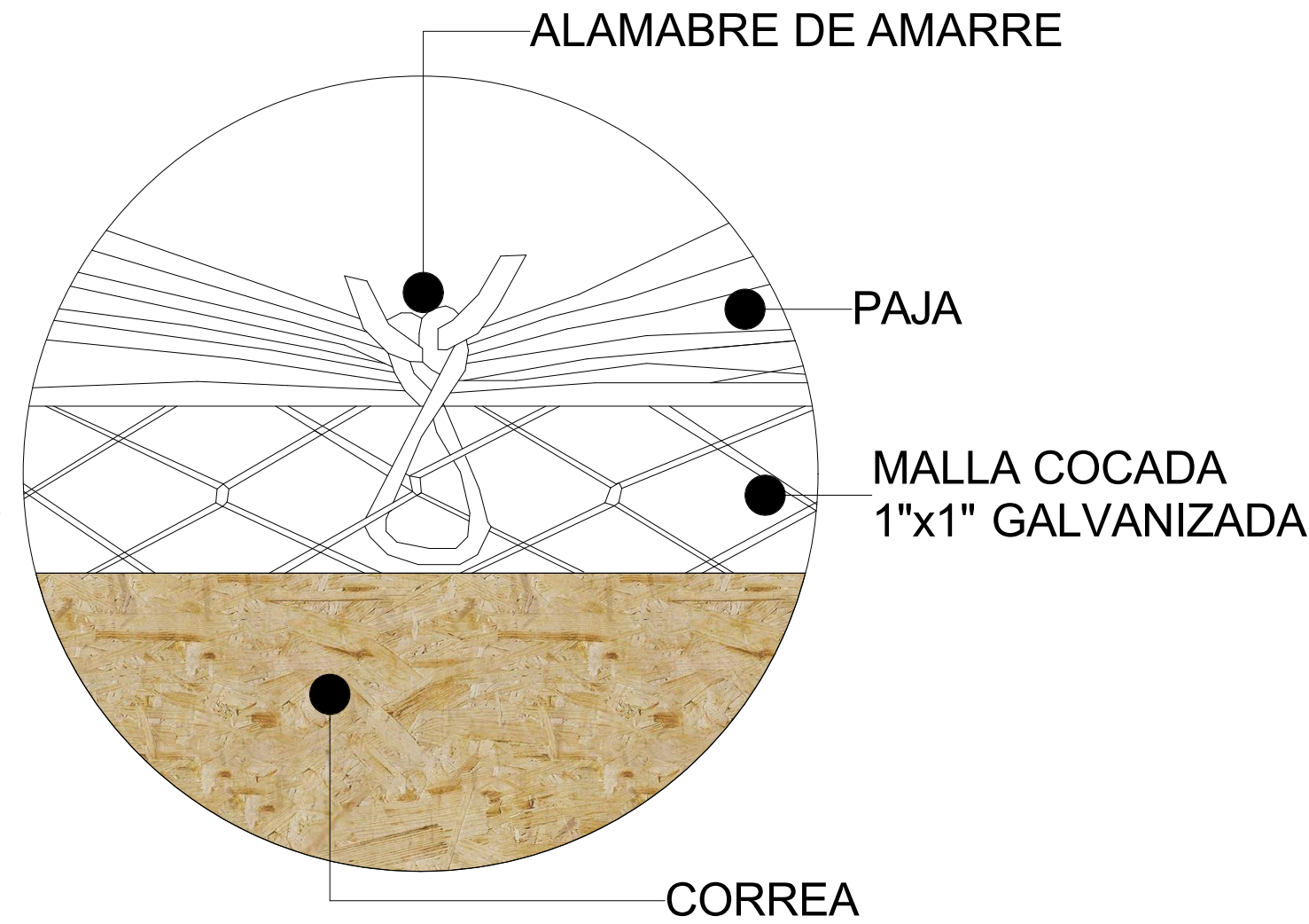
DETALLE AMARRE Y FIJACIÓN
