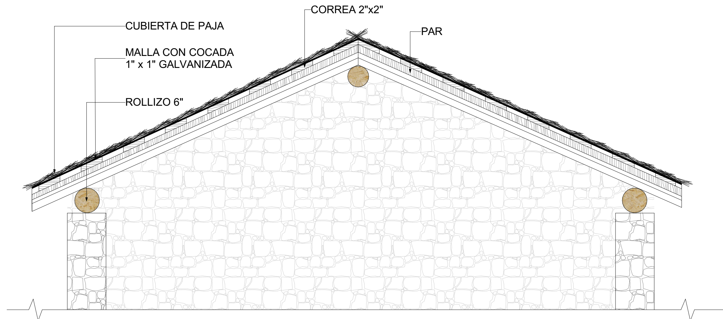
CORTE DE CUBIERTA
