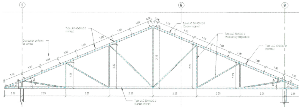
Tijeral tipo 1, 2 y 3
