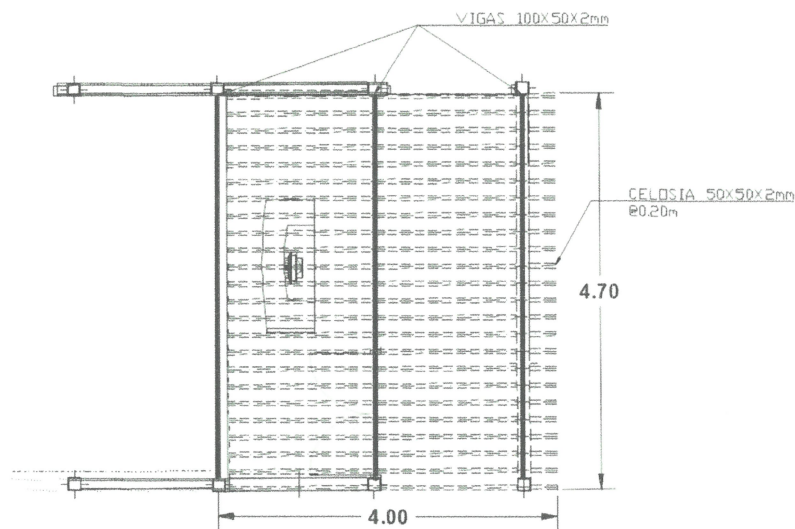
Detalle de celosía
