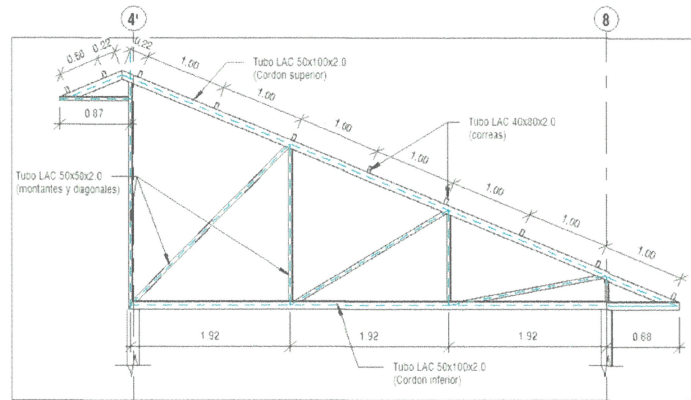
Tijeral tipo 4
