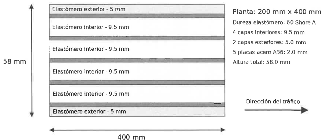
Figura 1. Esquema referencial del apoyo elastomérico laminado.
